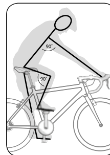
Kniewinkel oberes Bein min. 90°, Armwinkel 90°
