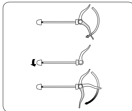
Einstellmutter anziehen
