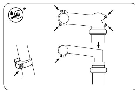
Mogelijke standen van boutverbindingen voor aanpassing
