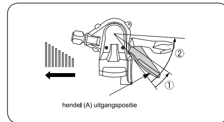
omschakelen van een kleine naar een groter tandwiel (hendel A)
