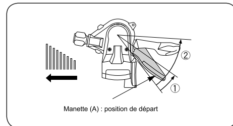
Passage d'un petit pignon à un grand pignon (manette A)
