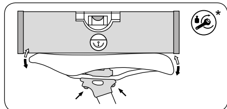
Tija con mecanismo de sujeción integrado con dos tornillos
