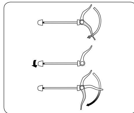
Einstellmutter anziehen
