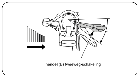
omschakelen van een groot naar een klein tandwiel (hendel B)
