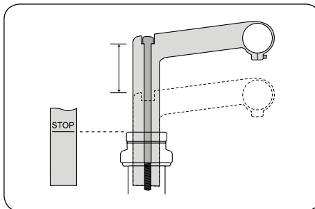
Regolabile in altezza
