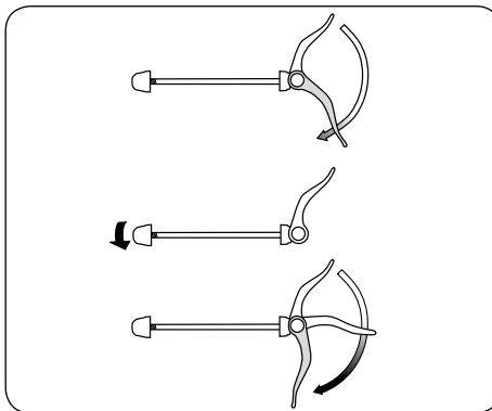
Serraggio del dado di regolazione
