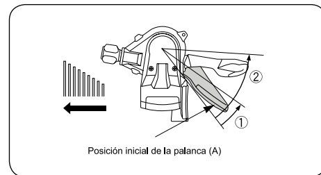
Cambio de un piñón pequeño a un piñón grande (palanca A)
