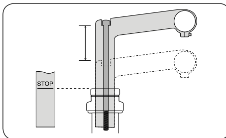
Altura regulable
