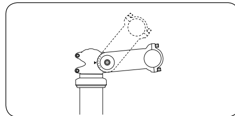
Possibile regolazione della pendenza del gambo
