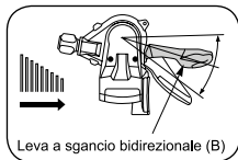
Cambio da un pignone posteriore più grande a uno più piccolo (leva B)
