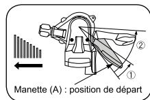
Manette (A) : position de départ Passage d'un petit pignon à un grand pignon (manette A)
