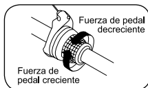
Cambio de un piñón grande a un piñón más pequeño (palanca B)
