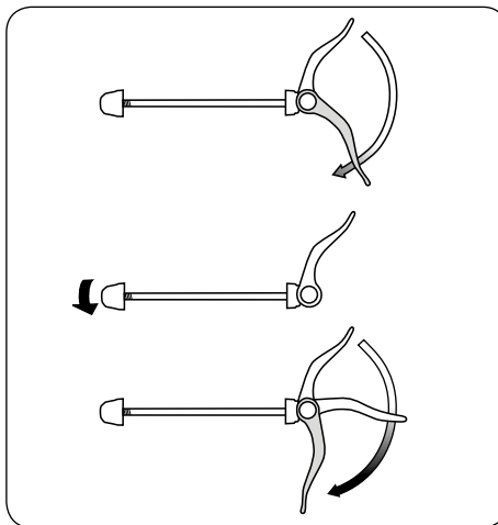
Apretar la tuerca de reglaje
