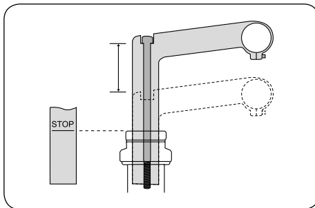
Höhenverstellung möglich
