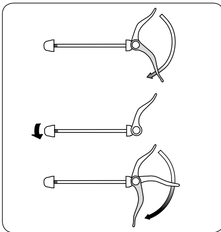
Einstellmutter anziehen
