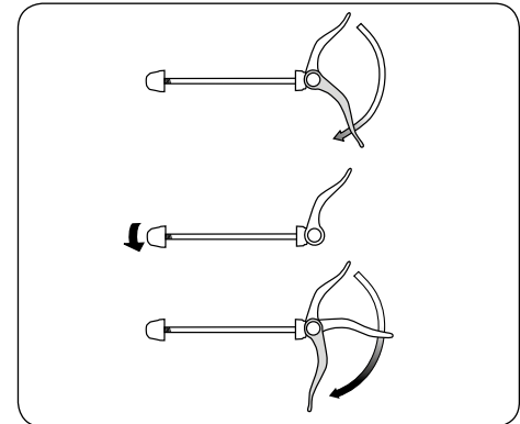
Einstellmutter anziehen
